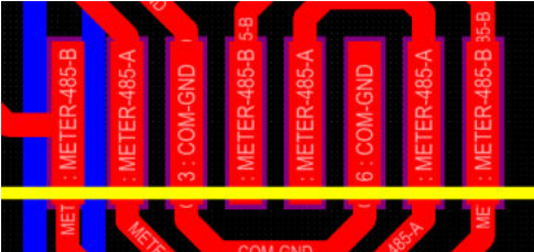
Contatore-Porta 485
