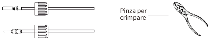
Fig. 3.4 Crimpare il pin di contatto sul filo
