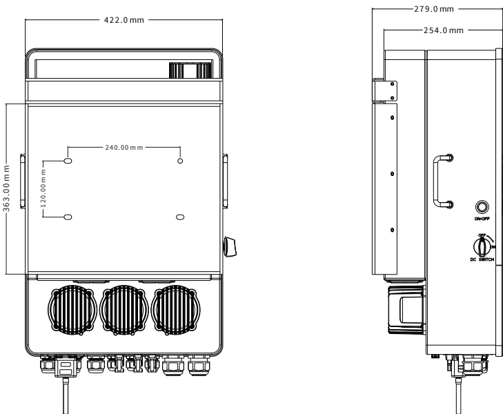
Dimensioni dell'inverter
