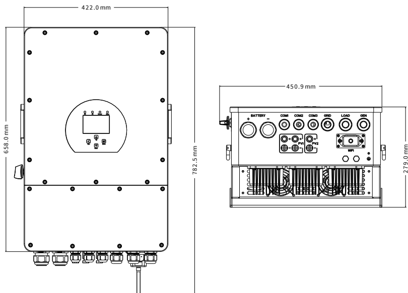
Dimensioni dell'inverter
